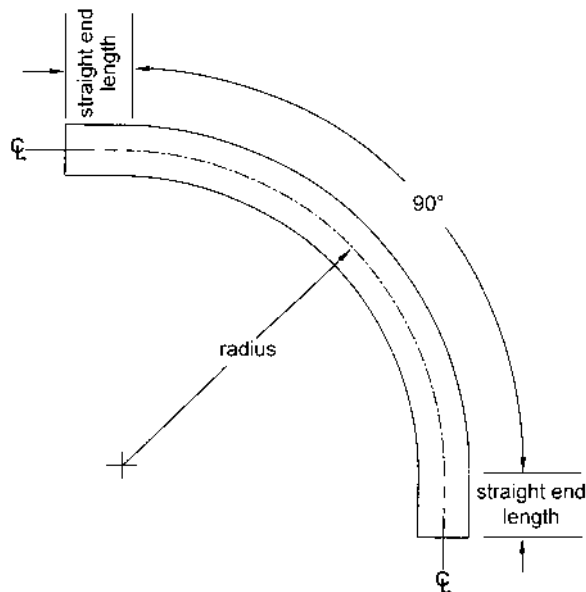
Figure 4.3a. Conduit Elbows
